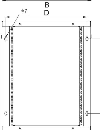
ВИД СЗАДИ
